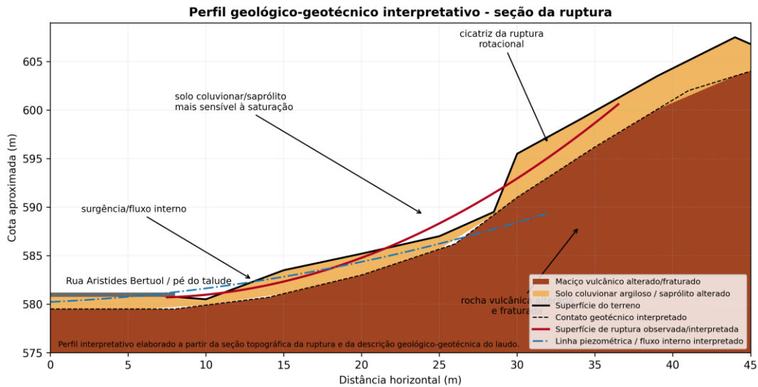
Figura 5. Perfil geológico-geotécnico interpretativo da seção da ruptura, com indicação dos dois materiais considerados na modelagem e da superfície de ruptura observada/interpretada.
